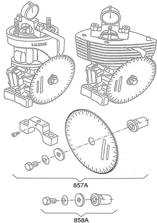
GRUPPO CONTROLLO FASE TIMING CONTROL GROUP GROUPE CONTROL DISTRIBUTION
