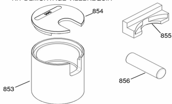
852A KIT SMONTAGGIO ALBERO CRANK DISASSEMBLING KIT KIT DEMONTAGE VILEBREQUIN
